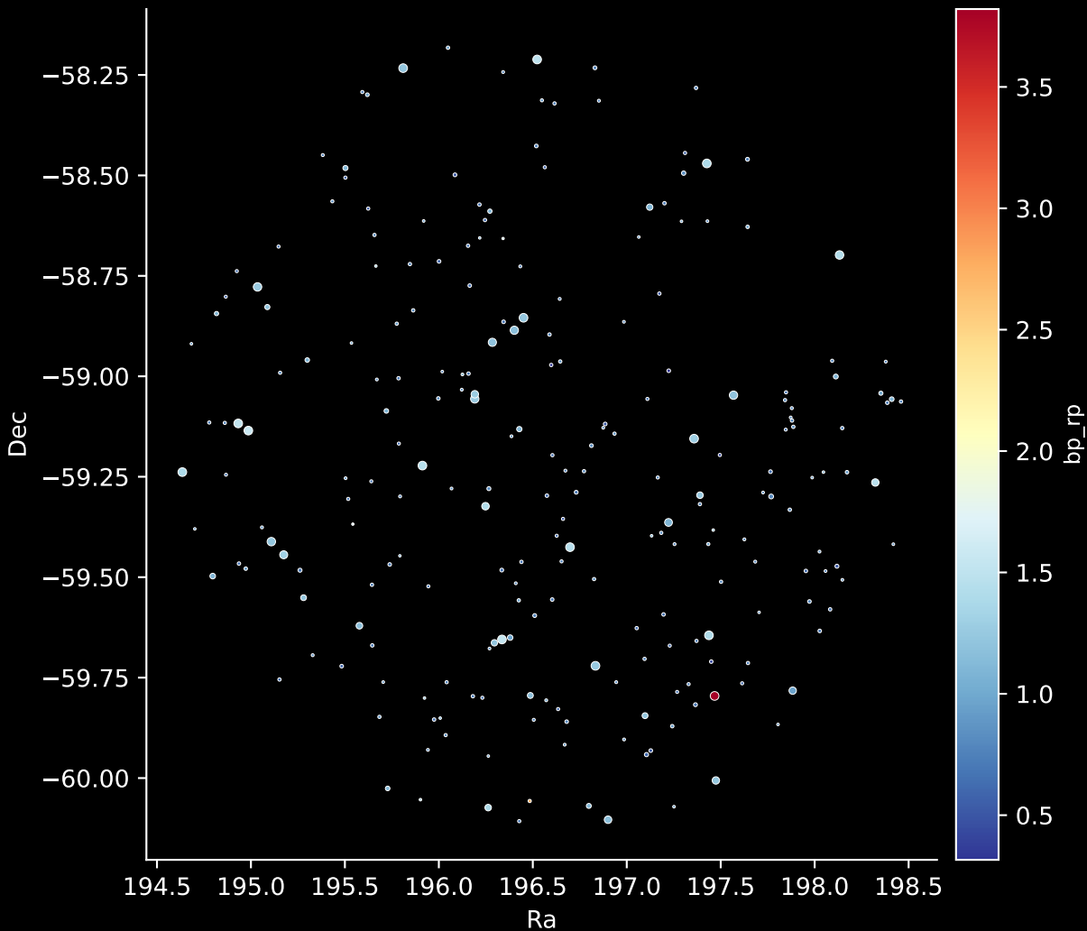
GALAH DR4 Field: [7162] Stars: 233
