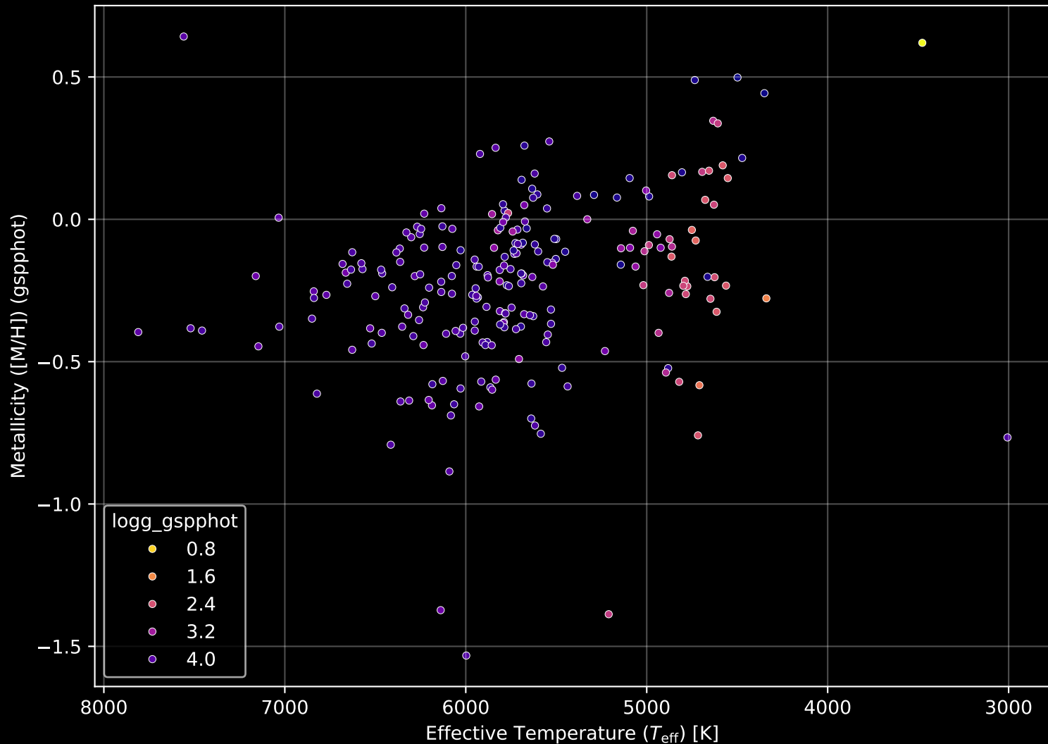
GALAH DR4 Field: [7162] Stellar Population Parameters (n= 233)
